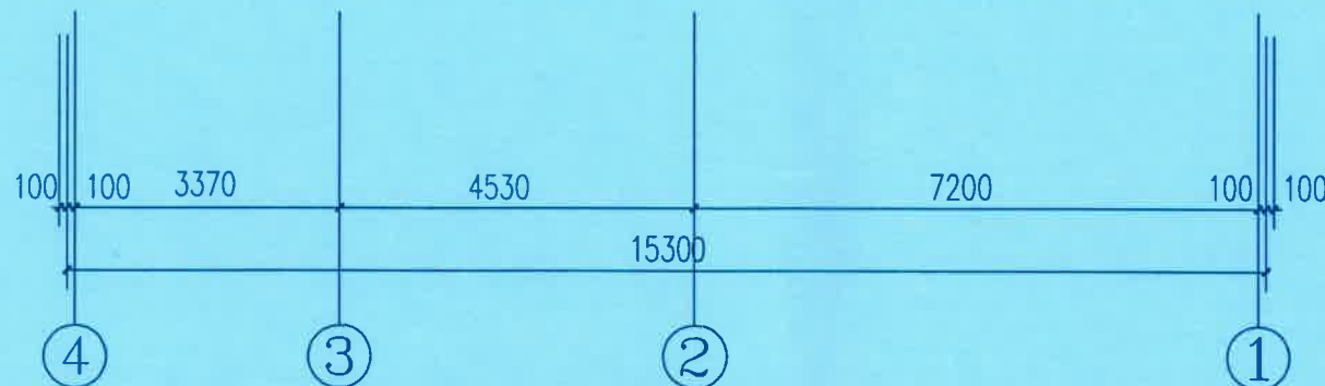
④~①轴立面图 1:100
