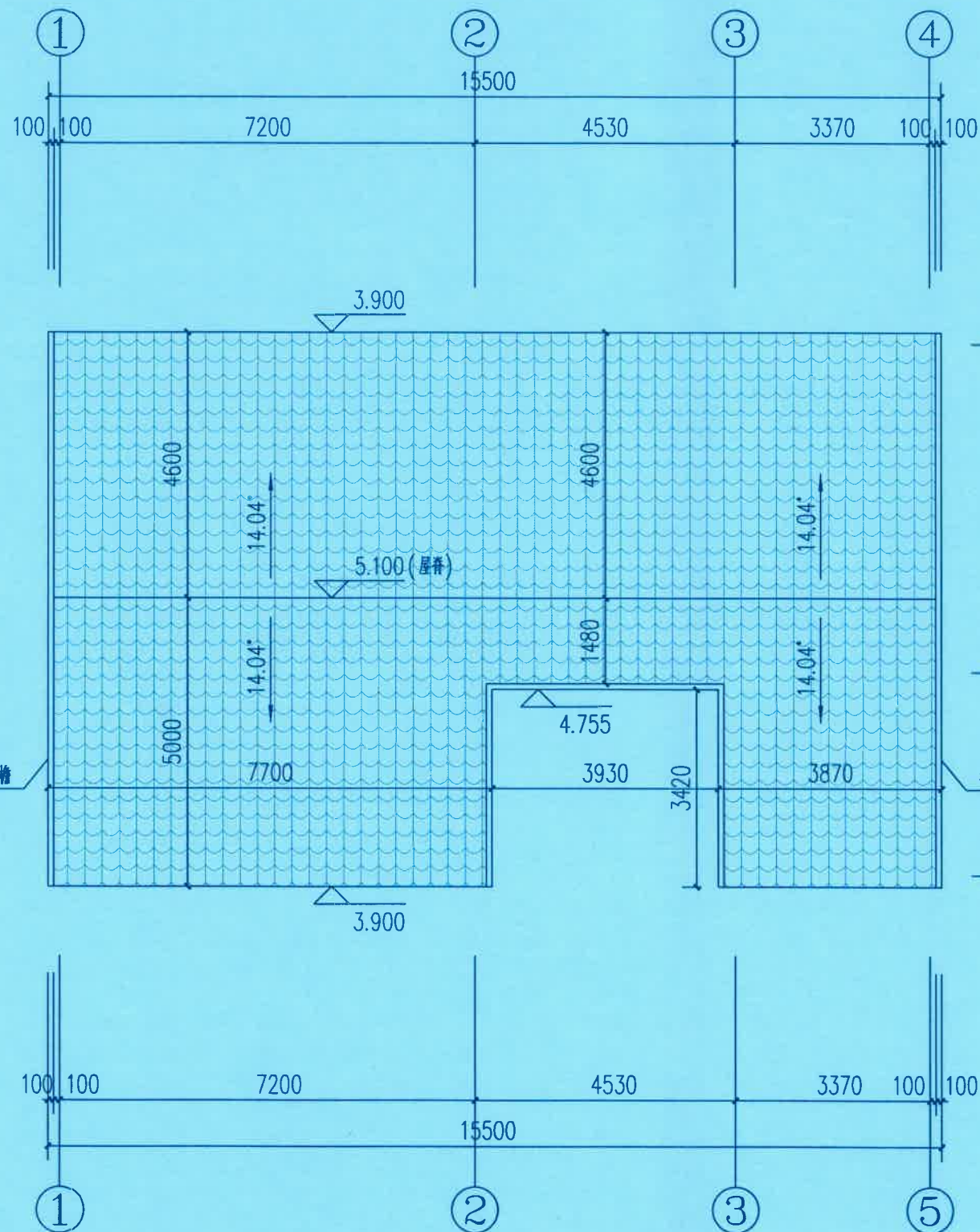
屋面层平面图 1:100
