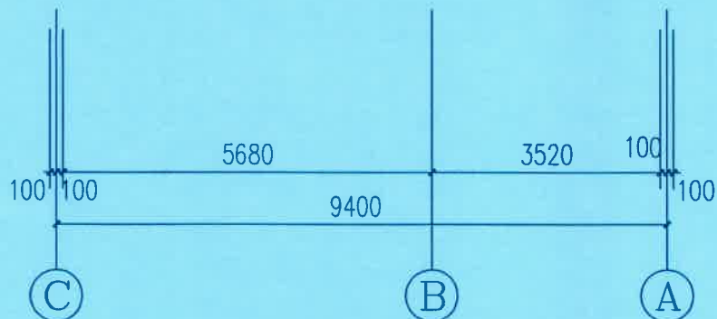
C~A轴立面图 1:100
