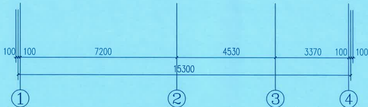
①~④轴立面图 1:100
