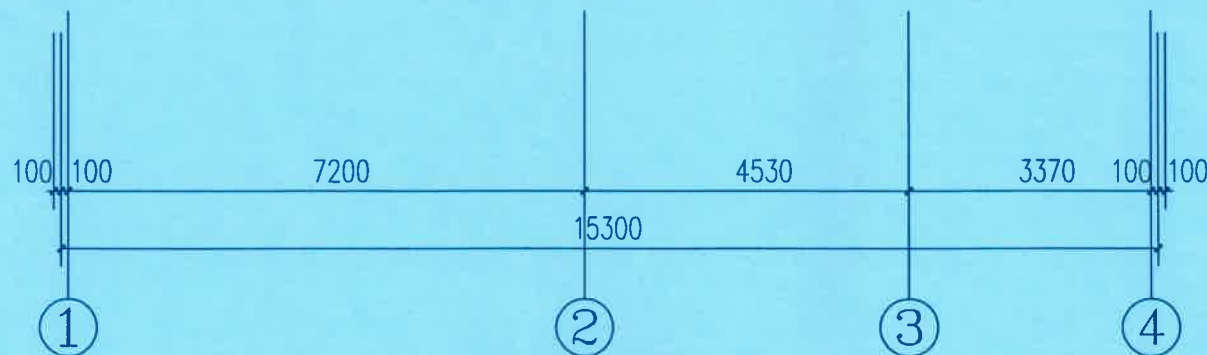
1-1剖面图 1:100
