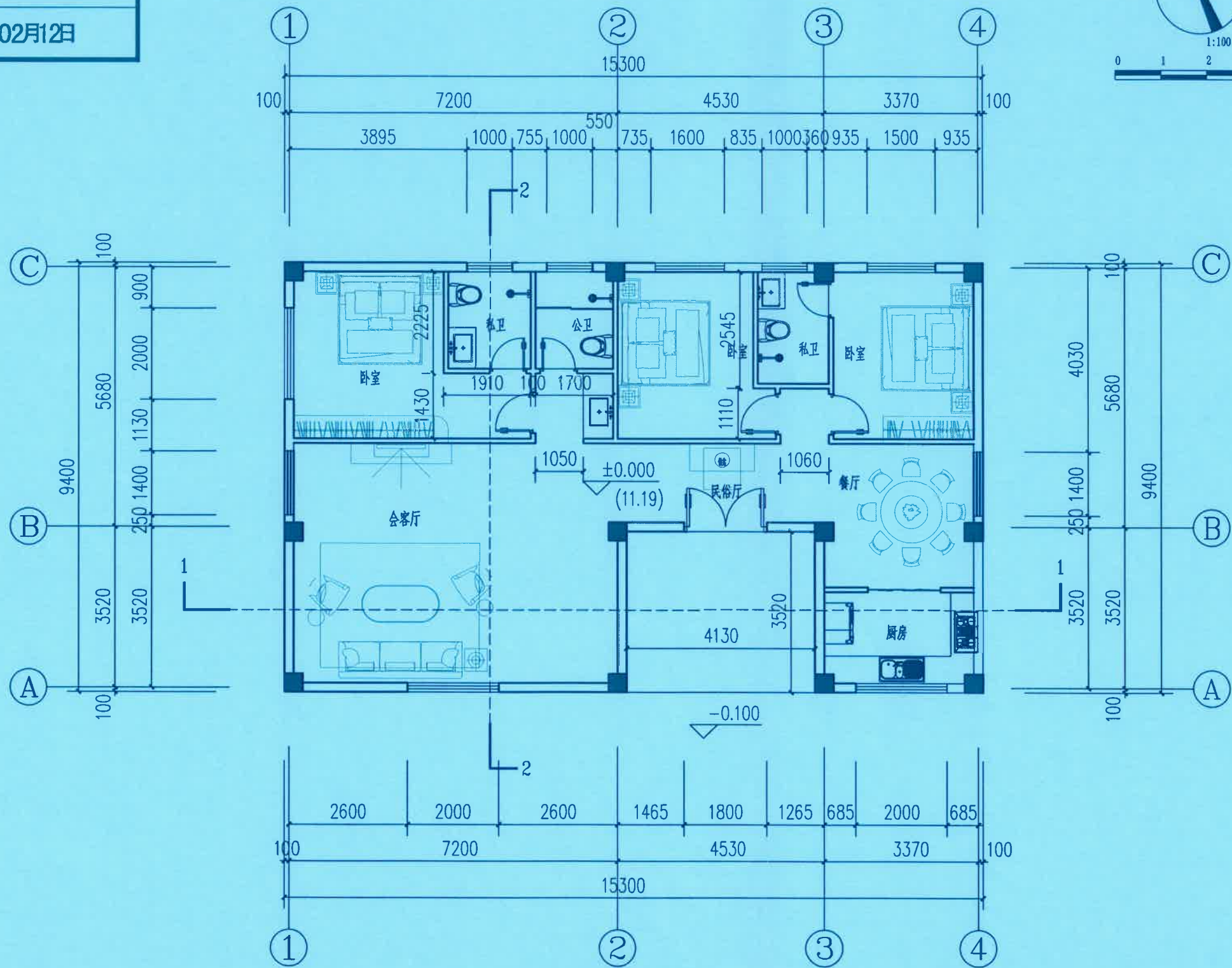
一层平面图 1:100
