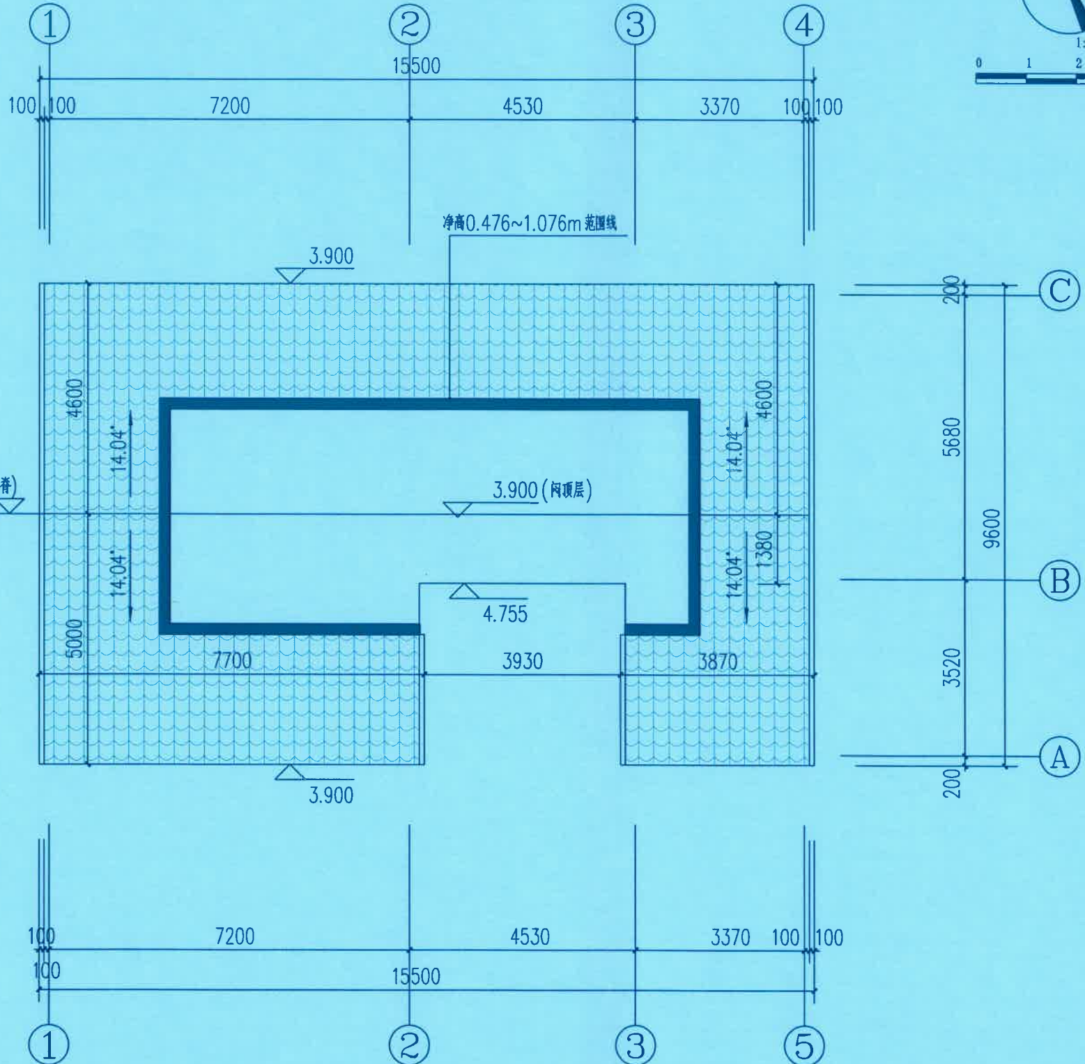
闷顶层平面图 1:100 本层建筑面积: 0 平方米(不计容)
