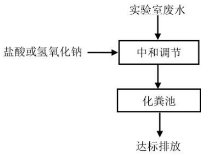
图 4-2 实验室废水处理工艺流程图
