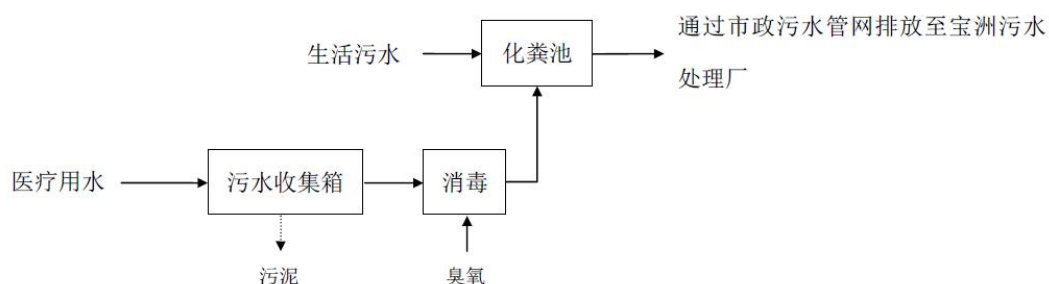
图 4-1 医疗废水处理工艺流程图
