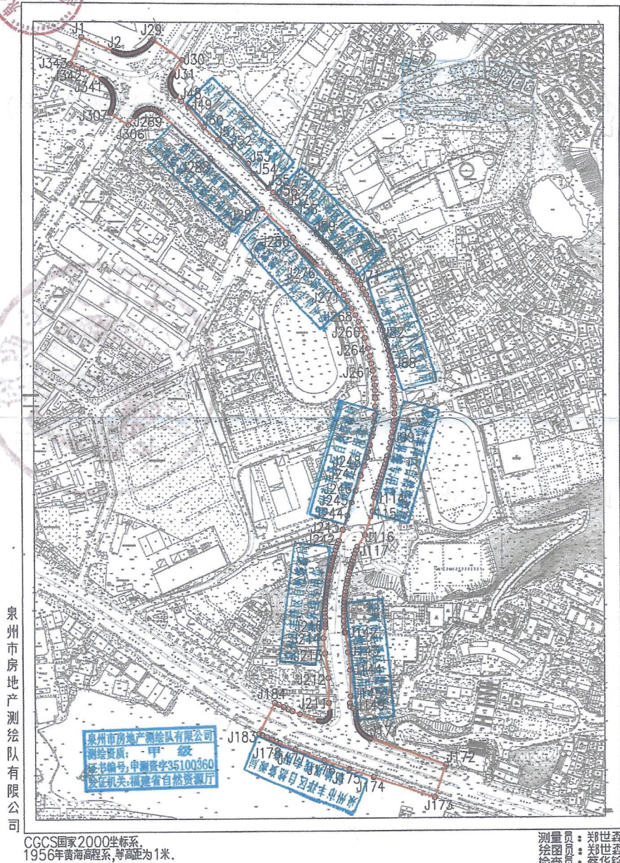
津淮街东延段工程（云鹿路至通港西街段）勘测定界图
