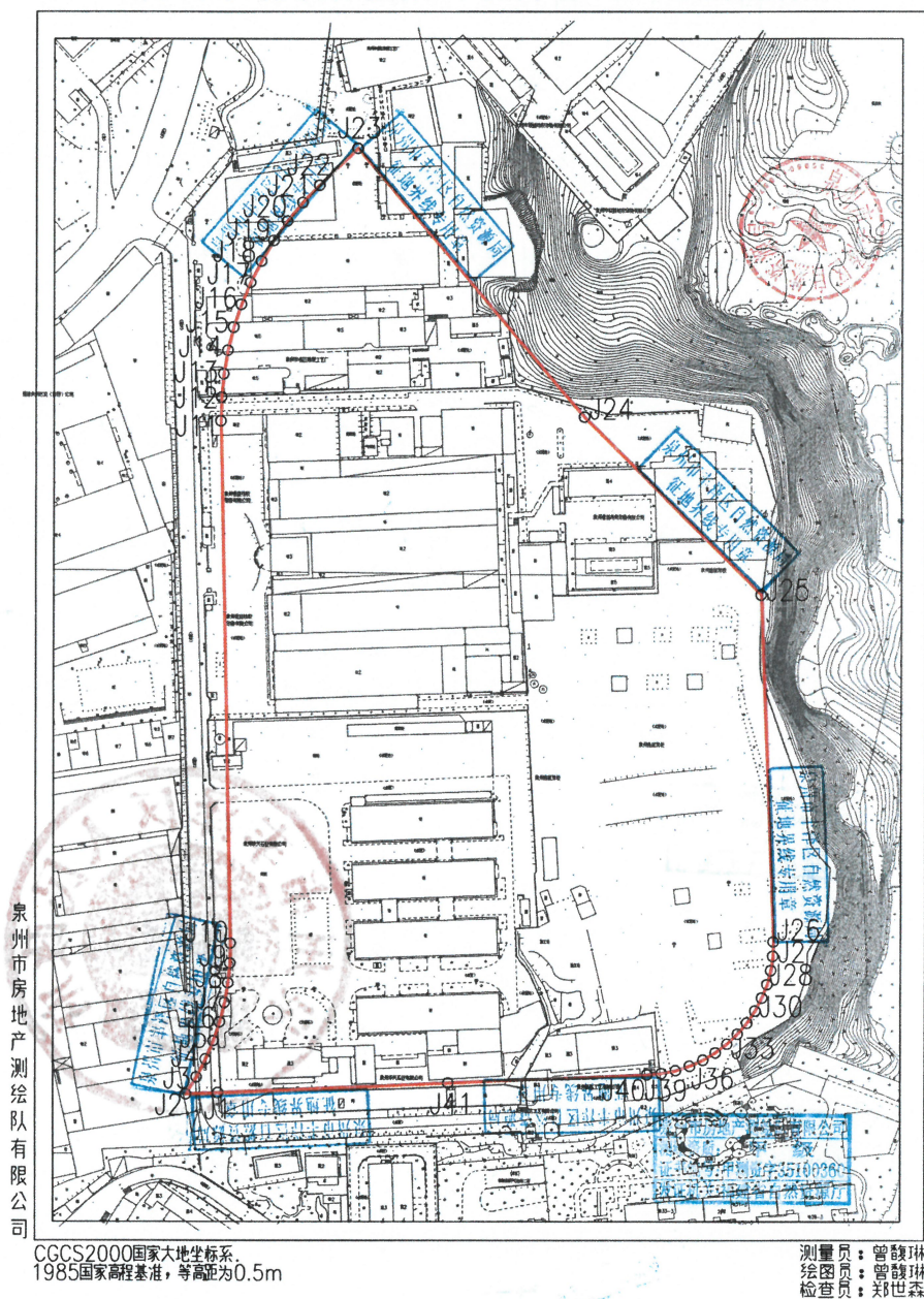
泉州市东海投资管理有限公司预申请工业用地勘测定界图
