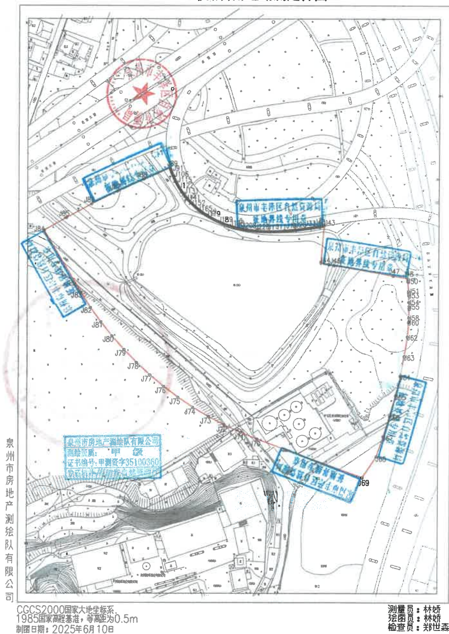
2025-13号储备用地勘测定界图
