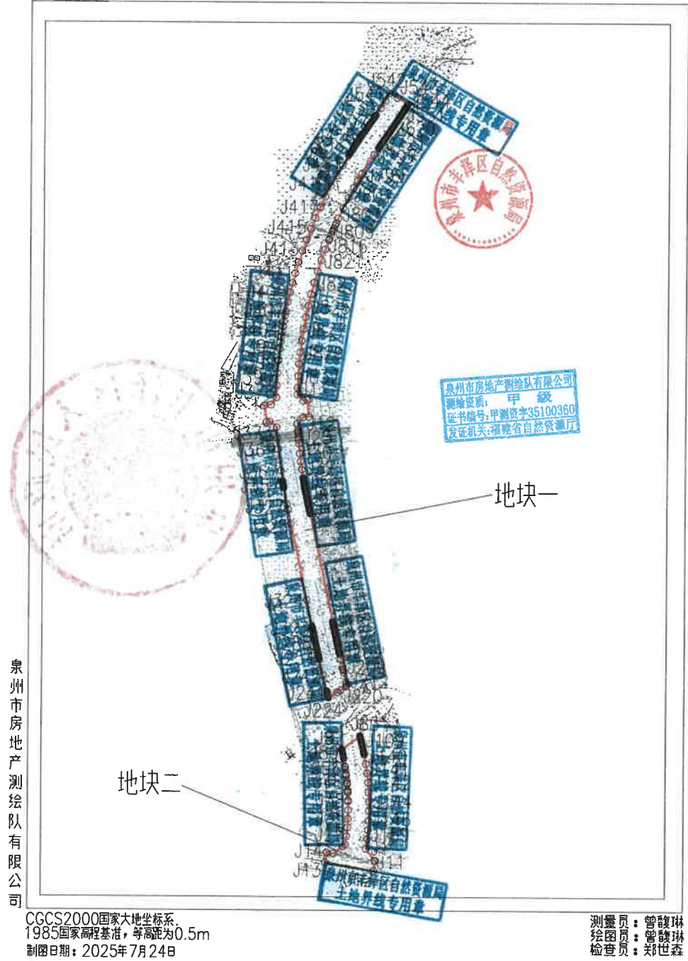
新华北路延伸段勘测定界图
