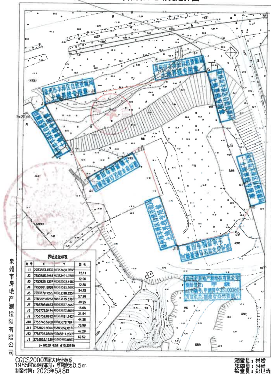
2024-9号储备用地勘测定界图
