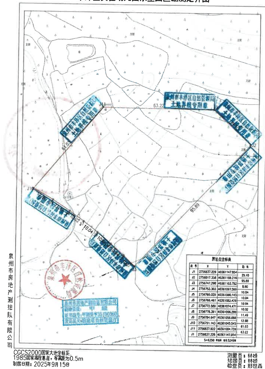
丰泽区实验幼儿园东星园区勘测定界图
